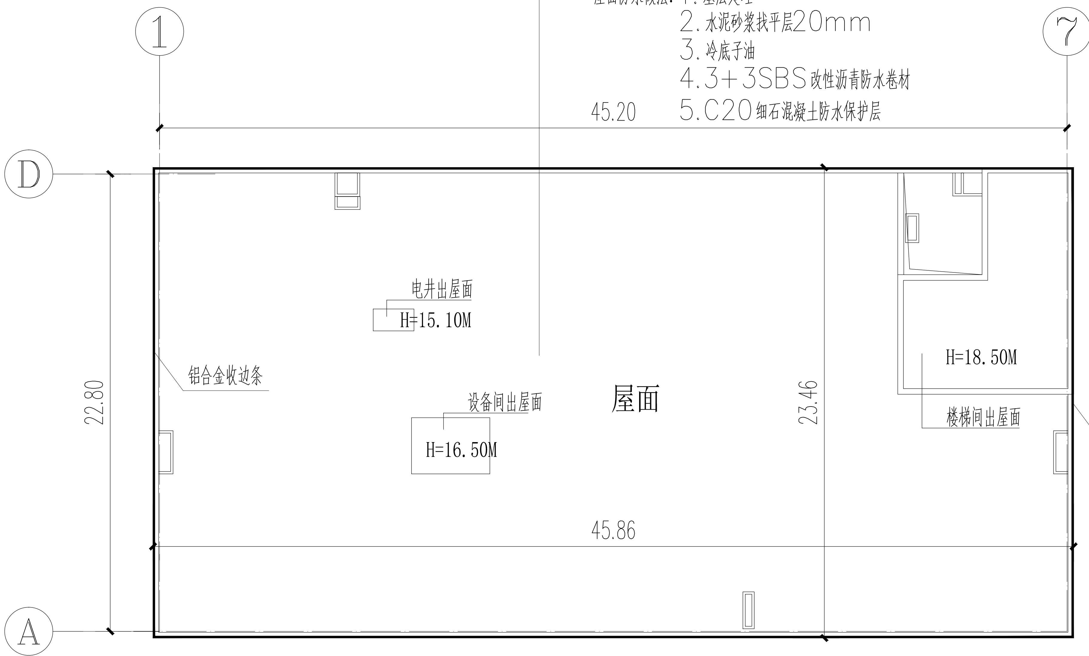
屋面平面图 1:300
