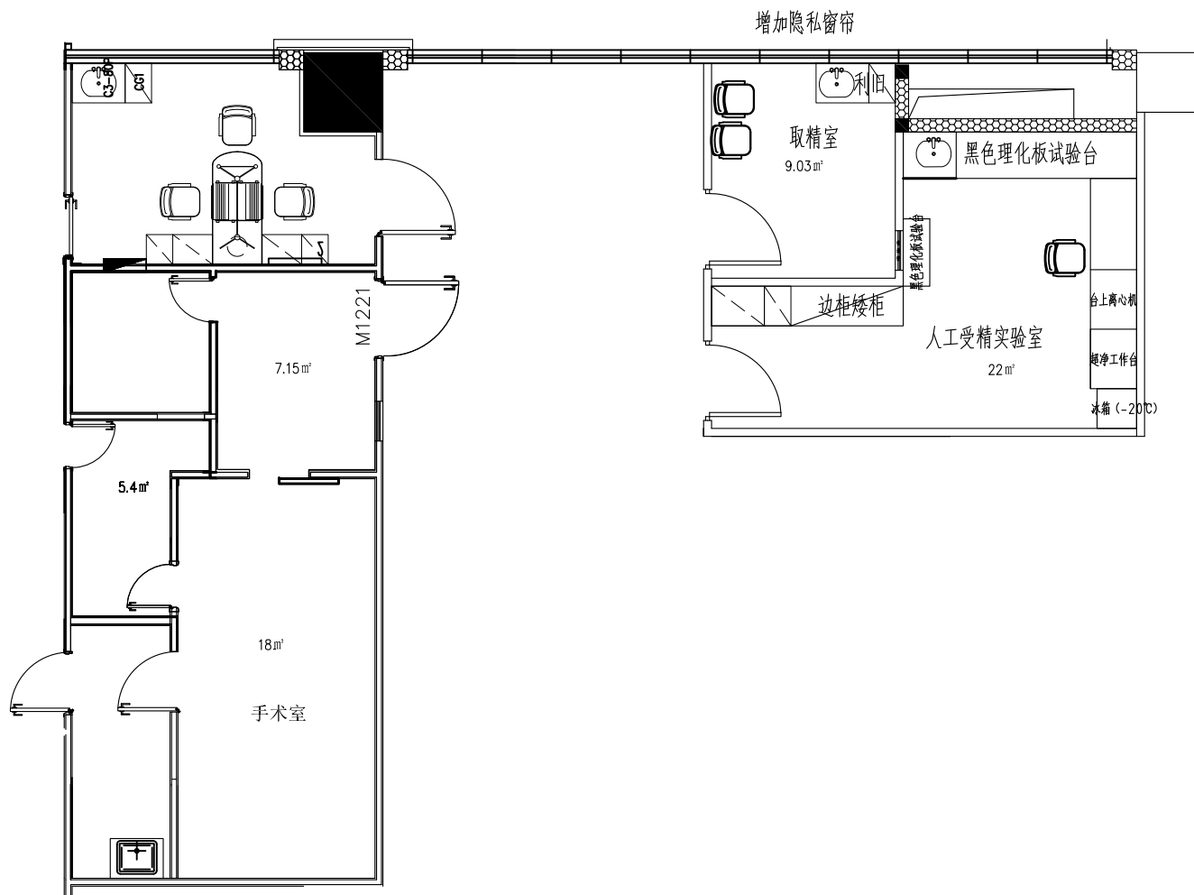
改造平面图
